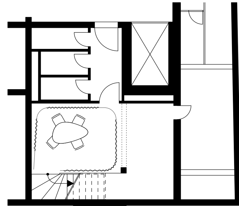
GRUNDRISS UG
